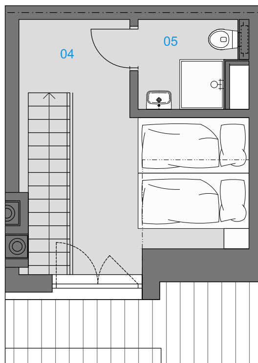
PŮDORYS PODKROVÍ
